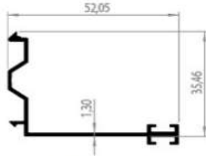
1330 - 0,407 kg/m KASA ÇITA-2
