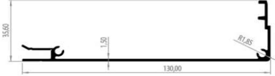
1317 - 0,870 kg/m MOTOR KASA PROFİLİ -1
