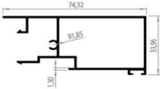
1328 - 0,827 kg/m BÜYÜK KAPAK PROFİLİ
